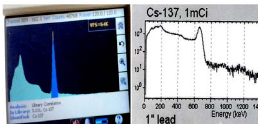
Figura 4. Espectro de muestra medida en forma experimental y Espectro de librería interna del equipo.
