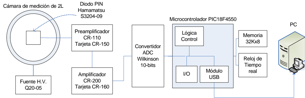
Figura 2. Diagrama de bloques general del prototipo RadonGuard desarrollado.
