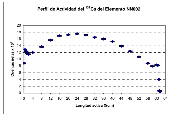
Figura 4: Perfil de actividad del ^{137}\text{Cs} para el Elemento Combustible NN002. El barrido se inició desde la boquilla del elemento combustible.
