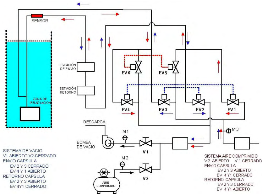
Figura 1: Representación esquemática del sistema neumático.
