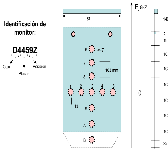
Figura 2: Esquemática de las dimensiones de la espada de aluminio, utilizada como portamuestra de los monitores metálicos, desnudos y bajo cadmio.
