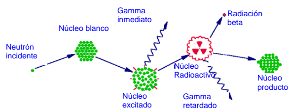
Figura 1: Proceso de interacción neutrónica y producción de gammas [1].
