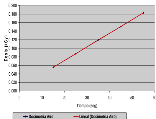
Grafico Nº 1 Linealidad de la Dosis Vs. Tiempo Equipo Gammacell 220-IPEN
