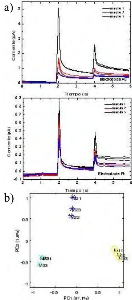
Figura 7: a) La respuesta de corriente en función del tiempo para las muestras de agua contaminada para los electrodos de Au y Pt, y b) la gráfica de componentes principales para el electrodo de Au.
