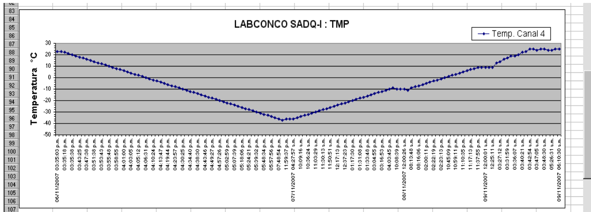
Figura 5: Gráfica de datos adquiridos por el canal 4 del sistema "Labconco SADQ-I".
