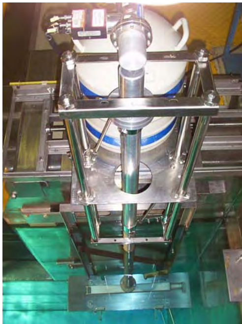
Figura 3: Disposición experimental del mecanismo de barrido.
