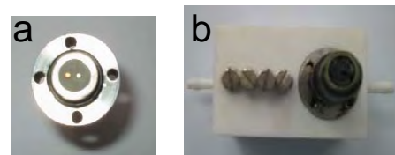
Figura 3: Fotografías de la parte superior del cabezal sensor (a) y de la cámara de medida (b).
