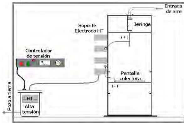
Figura 2: Diagrama experimental.
