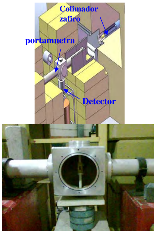
Figura 4: Arriba, esquema general de la instalación de facilidad, abajo fotografía de portamuestra de aluminio, con soporte de muestra y blindaje primario del detector de GeHP.
