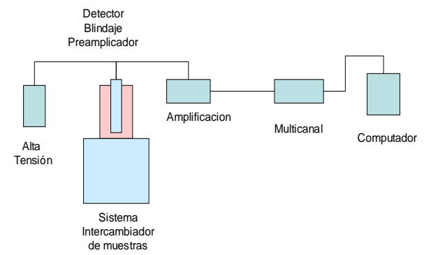
Figura 4: Esquema del equipo de medición utilizado.
