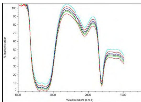
Figura 3: Perfiles de Espectros de gel de Aloe vera irradiado a 0, 5, 8, y 15 KGy. Pico de absorción: 1631\text{ cm}^{-1} .
