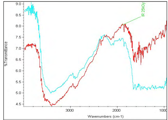
Figura 3: Comparación de los Espectros de las muestras de Rutina, control 0kGy y de la irradiada a la dosis máxima de 25 kGy.
