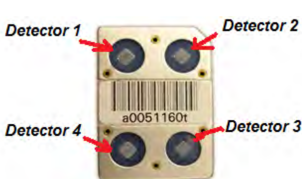
Figura 2. Tarjeta TLD tipo 7776 [3].
