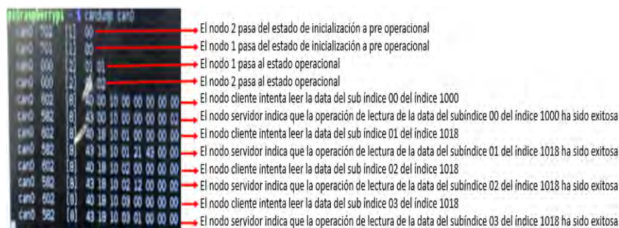
Figura 4. Mensajes CANOpen obtenidos mediante el comando candump .
