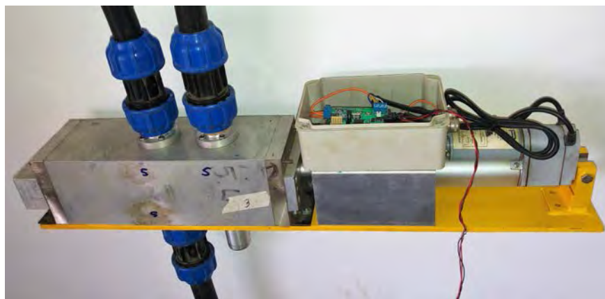
Figura 8. Actuador lineal encargado cambiar el recorrido de las muestras.
