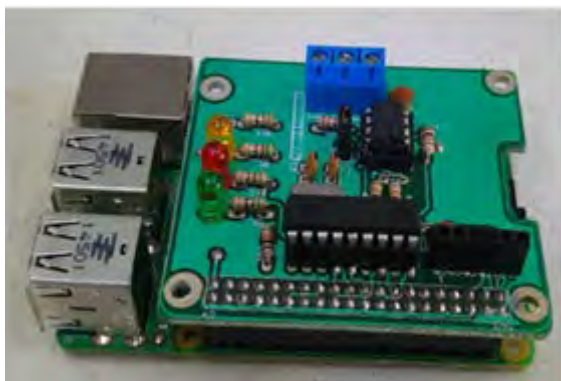
Figura 2. Tarjeta PICAN adaptada para ser usada en el Sistema Intercambiador de Muestras y montada sobre un Raspberry PI 2.
