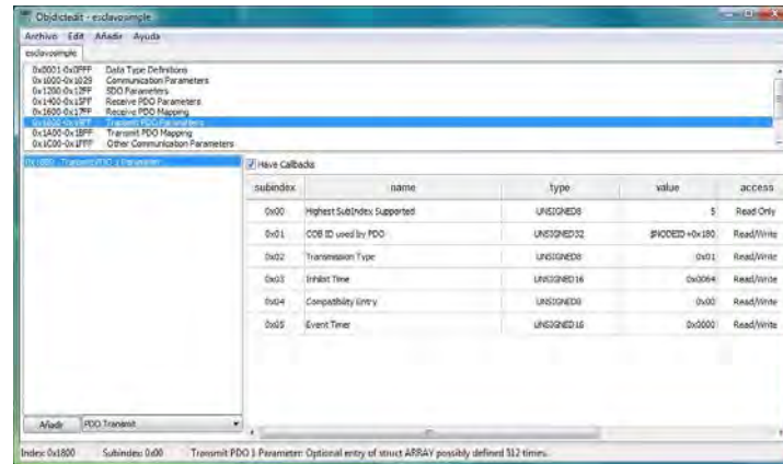
Figura 5. Editor de diccionario de objetos esclavo simple.od.
