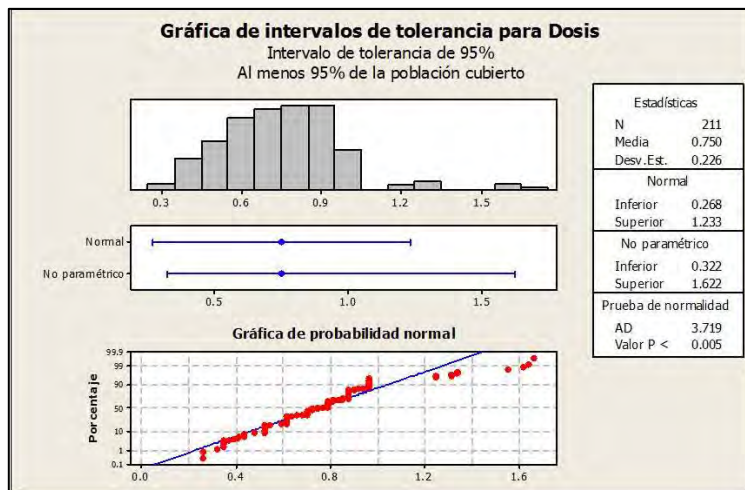
Figura 2. Equivalente de Dosis Ambiental en suelo superficial.
