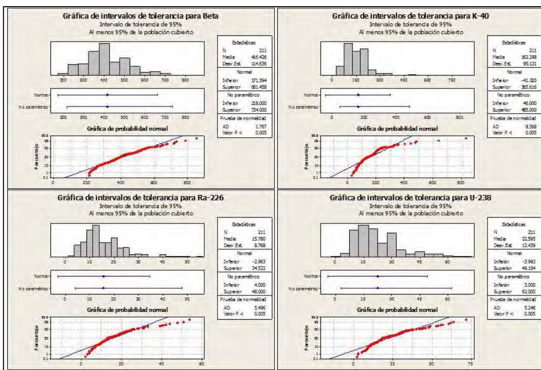
Figura 3. Niveles Beta Total, K-40, Ra-226 y U-238 en suelo superficial.
