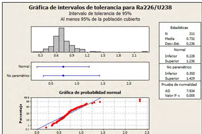
Figura 5. Índice Ra-226/U-238 en suelo superficial.
